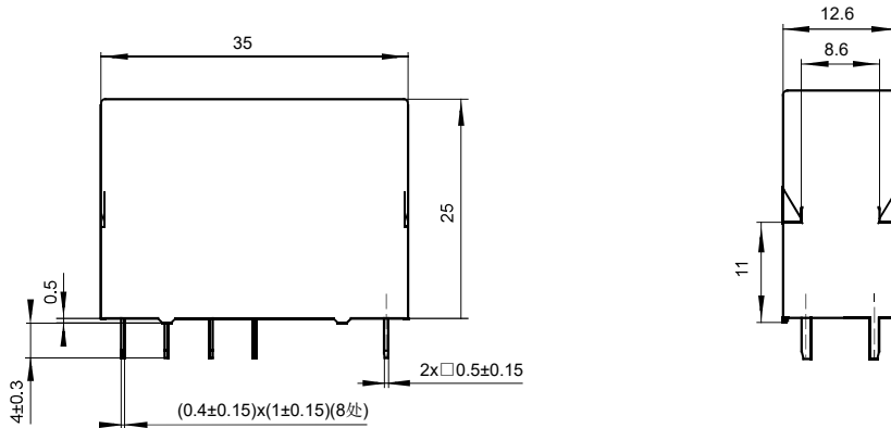
外形图
